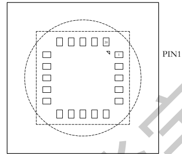
底部示意图
